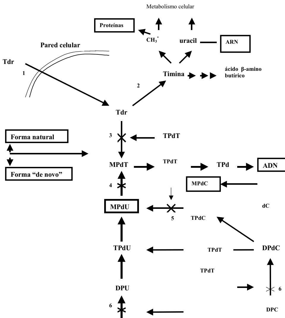
Figura 1. Caminos metabólicos del nucleótido timidina: Tdr , timidina; MPdT , DPdT y TPdT , timidina mono, di y trifosfato respectivamente; MPdU , DPdU y TPdU , desoxiuridina mono, di y trifosfato respectivamente; dC , desoxicitidina; MPdC , DPdC y TPdC , desoxicitidina mono, di y trifosfato respectivamente. Enzimas: (1) mecanismo de transporte activo; (2) timidina fosforilasa; (3) timidina quinasa; (4) timidilato sintetasa; (5) desoxicitidilato deaminasa; (6) ribonucleosido reductasa.
