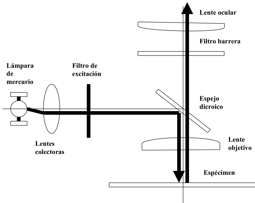
Figura 1: Esquema del camino que sigue la luz (camino óptico) de un microscopio de fluorescencia convencional, donde se puede apreciar la ubicación de los filtros de barrera y excitación.
